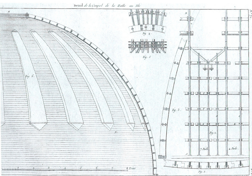
Halle au blé, Paris, Kuppel 1783. Querschnitt (aus: M. K. Deming, wie Anm. 12) und Konstruktionsschnitt (aus: J. Ch. Krafft, Plans, coupes et élévations [...], Paris 1805; ETH Zürich, Sammlung Alte Drucke)
